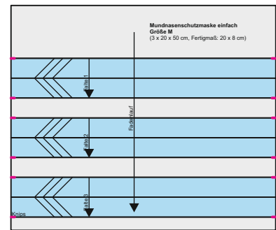
Mundnasenschutzmaske, Schnittteil
